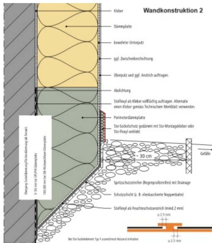
Wandkonstruktion 2
