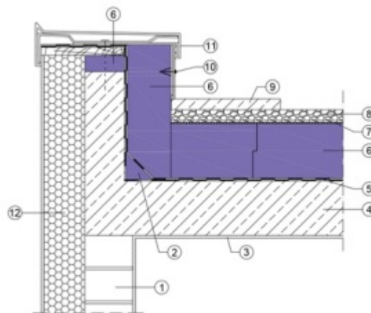
Dachkonstruktion 2
